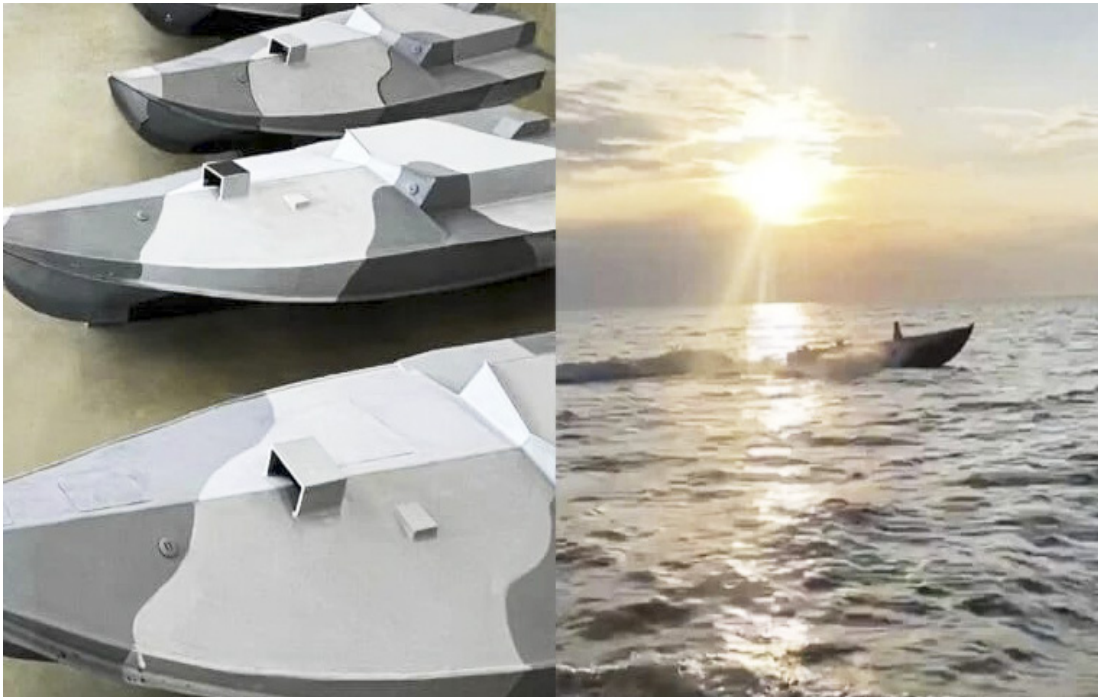
Člny sú vybavené autopilotom aj systémom nočného videnia.
